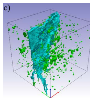
Trójwymiarowa struktura betonu: a) nieprzetworzone dane z mikro-tomografii komputerowej, rekonstrukcja: b) kruszywa oraz c) pęknięć (niebieski) i porów powietrznych (zielony)
